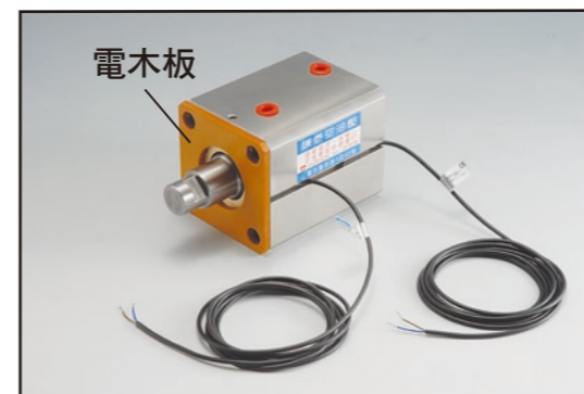
電木板 模具溫度超過80°C以上，建議模具與油壓缸間加電木板隔離溫度，電木板厚5mm
